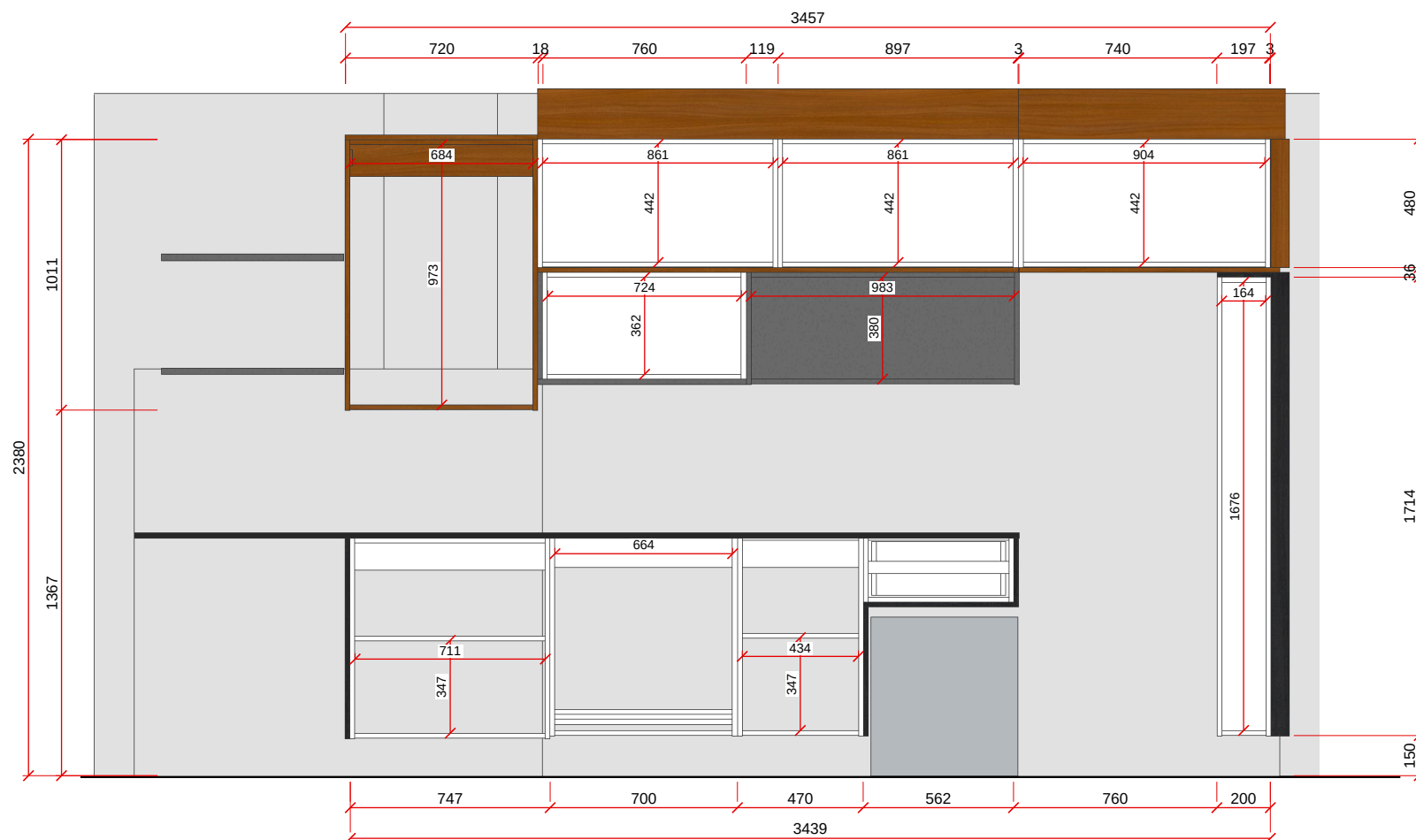
VISTA A - ESC. 1:25
